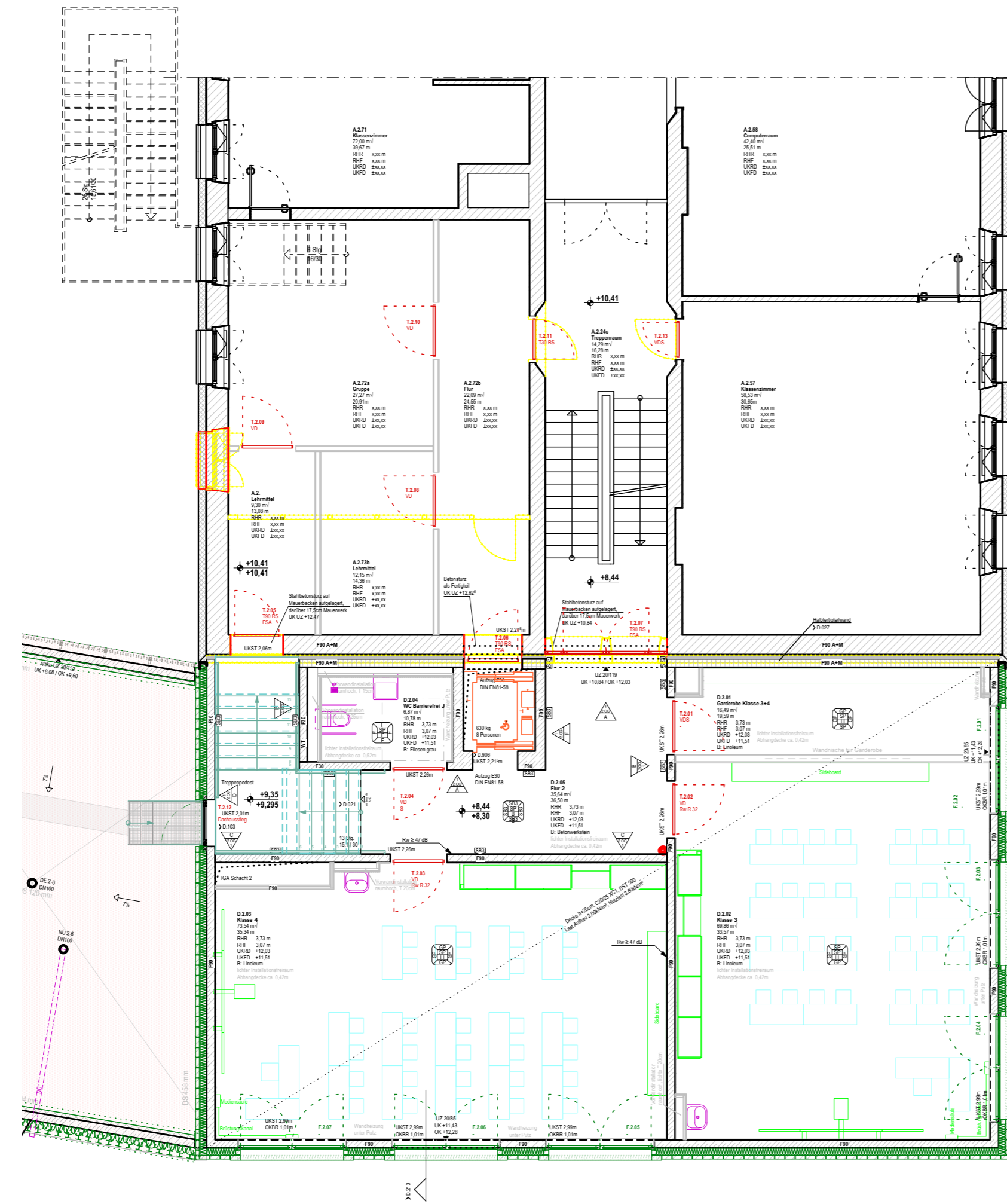
GRUNDRISS 2. OBERGESCHOSS
