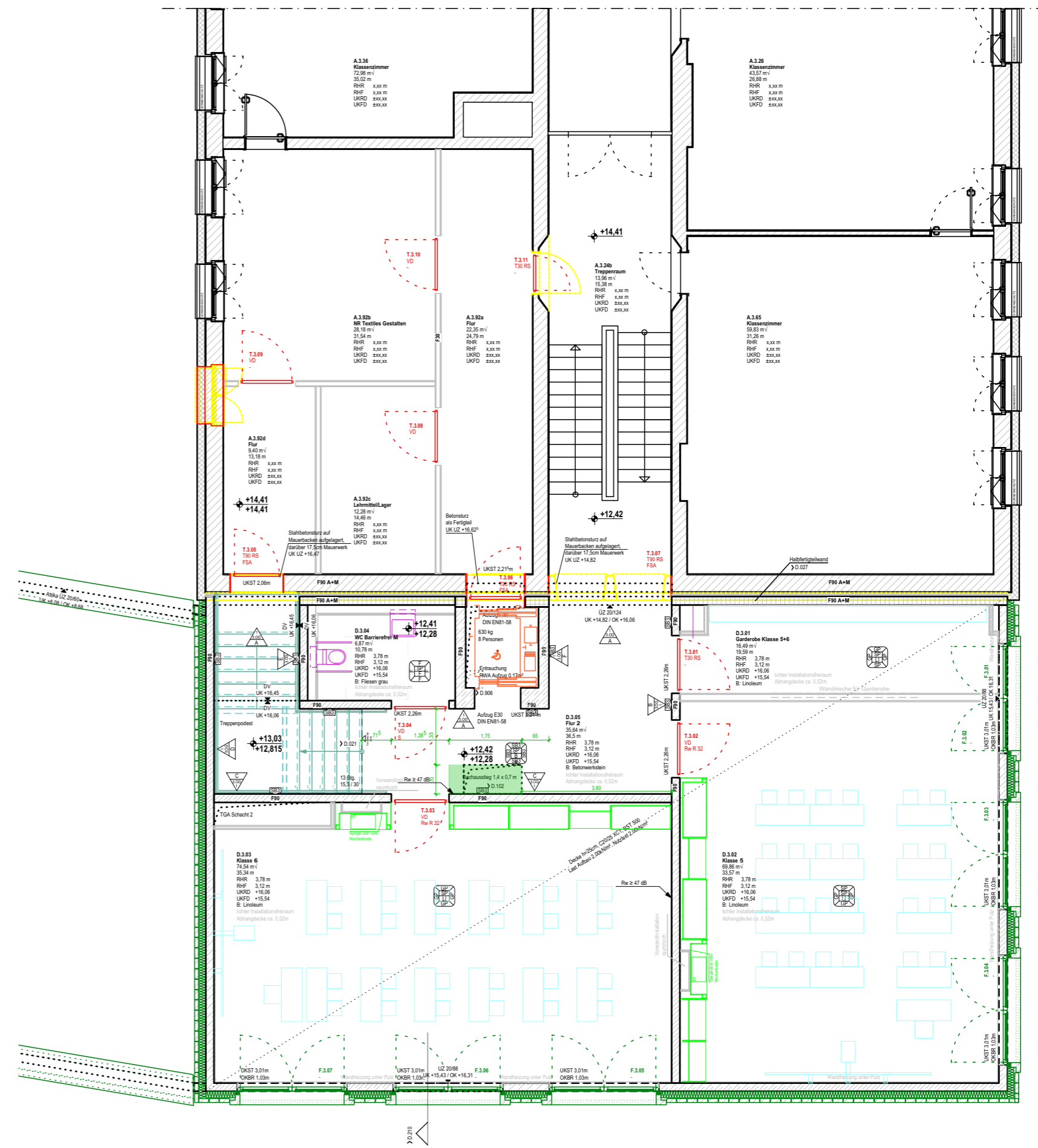
GRUNDRISS 3. OBERGESCHOSS
